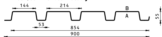
TRB-55K/854 Profil odwracalny
