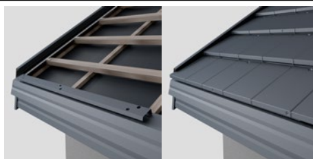
Listwa startowa wentylacyjna LSW Garda
